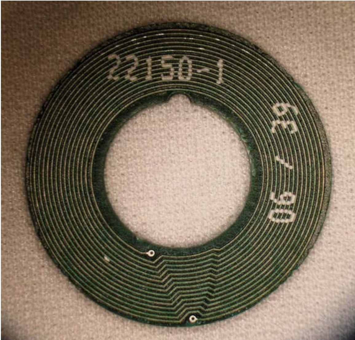
RFID Tag Bottom
