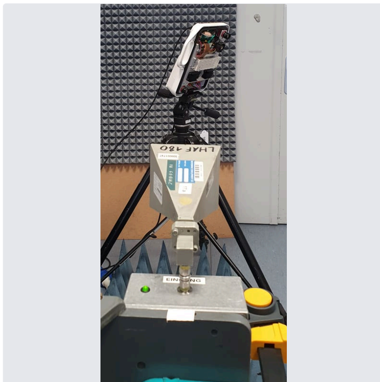
Photo 7 EUT 1
