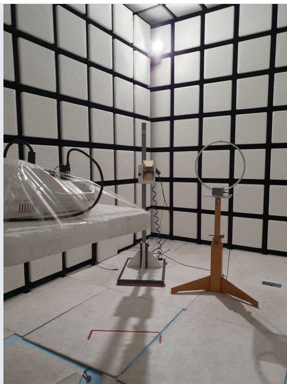
Photo 5 EUT 1
