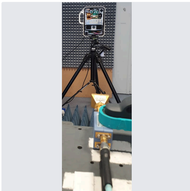
Photo 6 EUT 1
