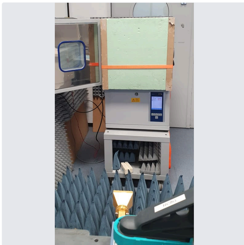
Photo 8 EUT 1
