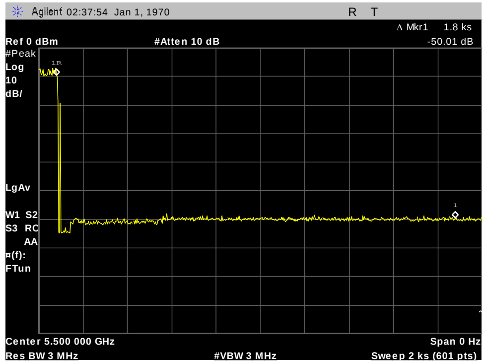
Figure 41: 5500 MHz Non Occupancy
