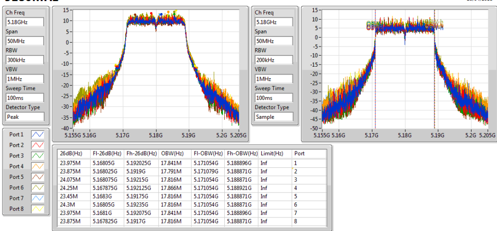
802.11ac VHT20-BF_Nss1,(MCS0)_8TX
