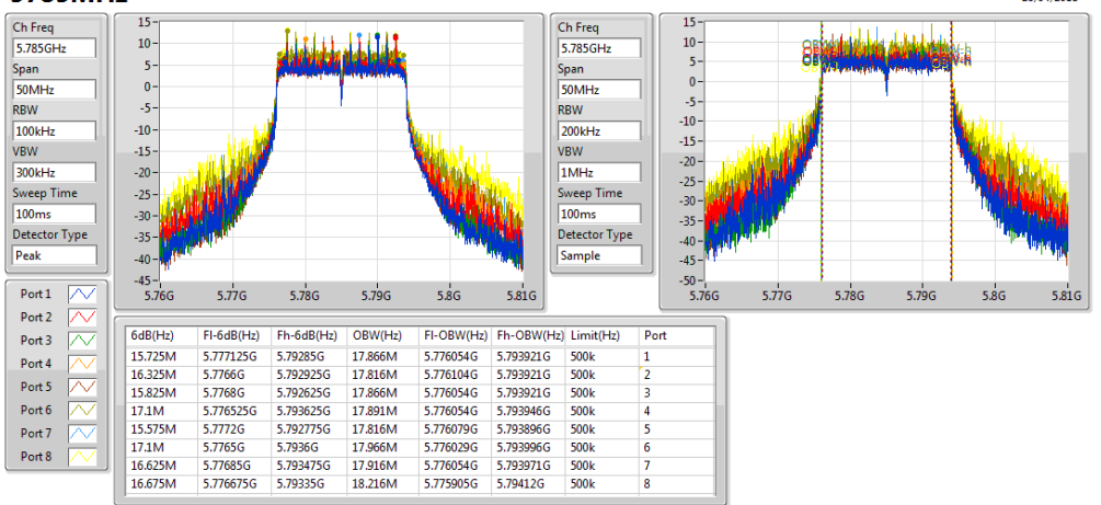
802.11ac VHT20-BF_Nss1,(MCS0)_8TX
