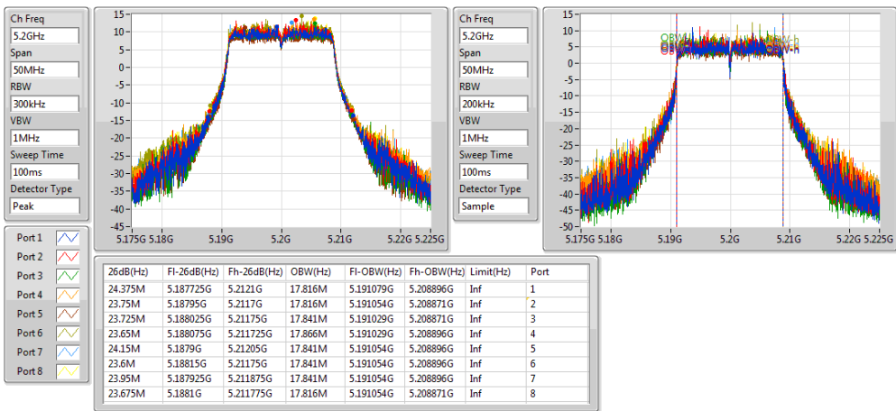
802.11ac VHT20-BF_Nss1,(MCS0)_8TX
