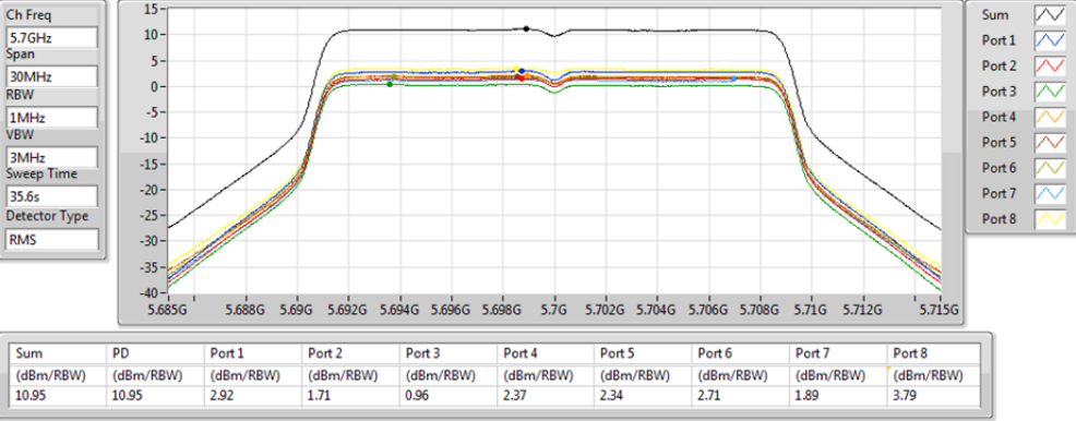
802.11ac VHT20-BF_Nss1,(MCS0)_8TX
