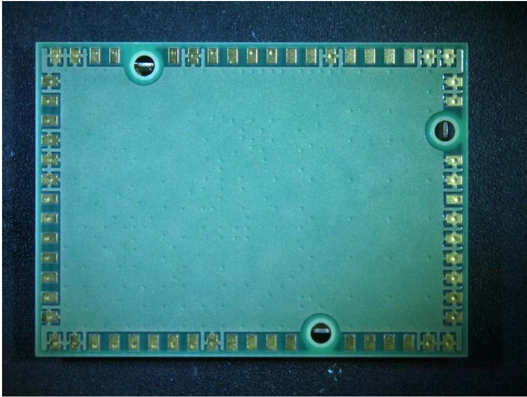
Radio Module
