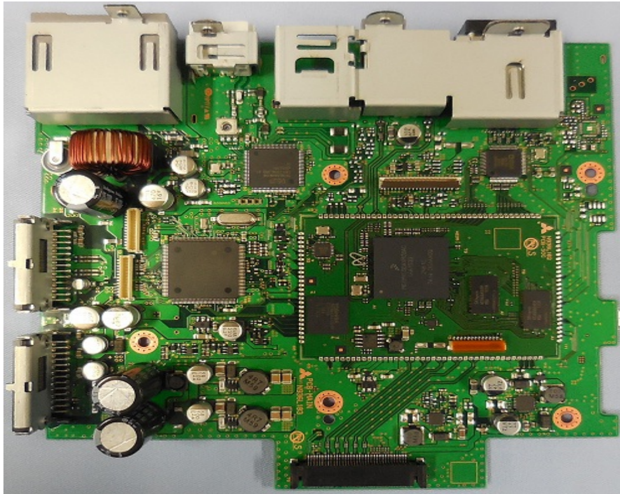
1. PCB-NAVI C-side
