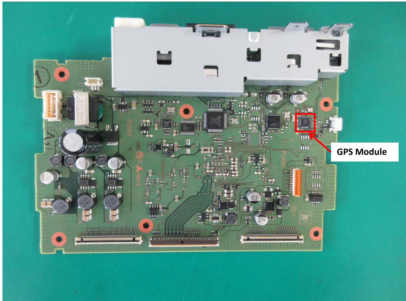
1. PCB-NAVI C-side
