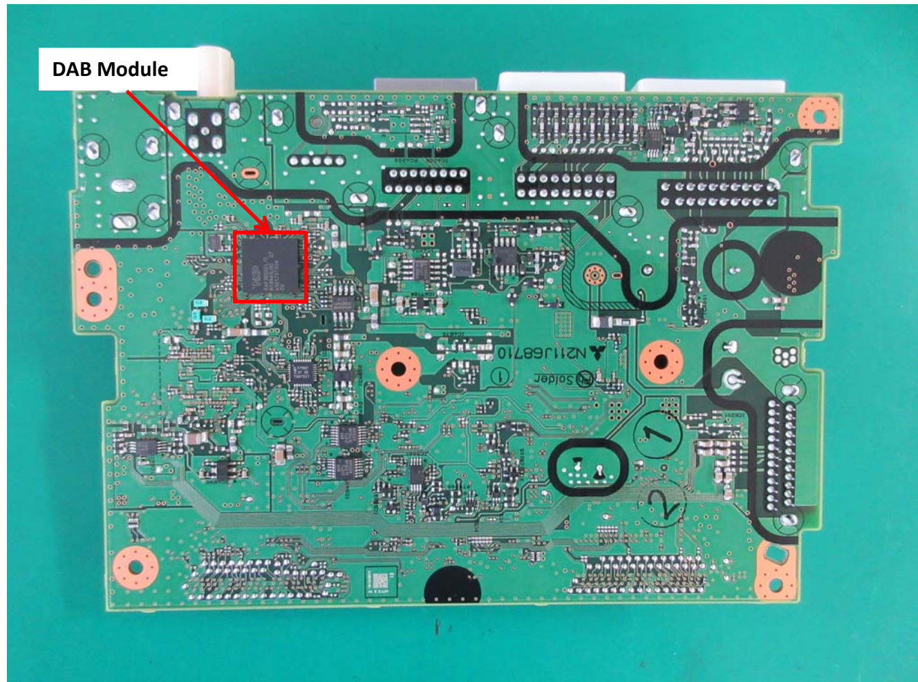
4. PCB-AUDIO S-side
