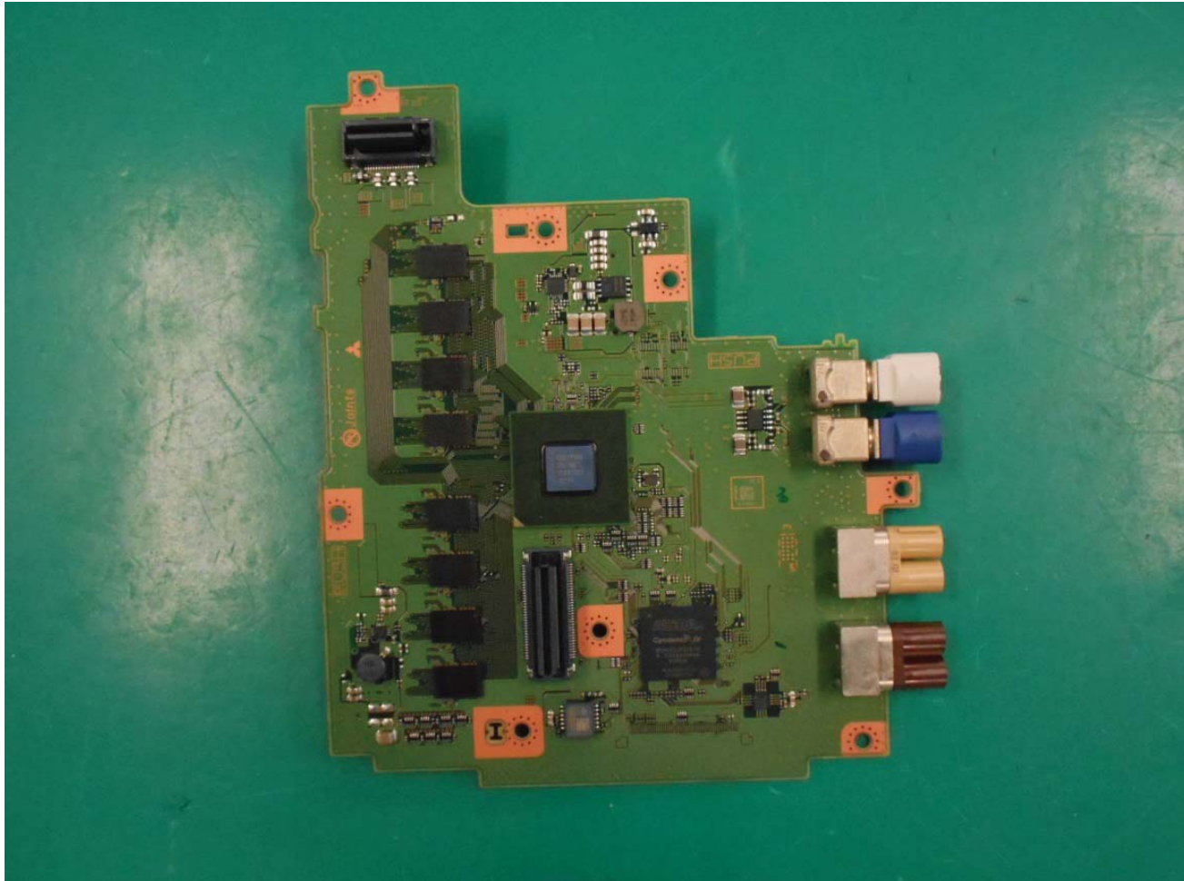
1. PCB-NAVI C-side
