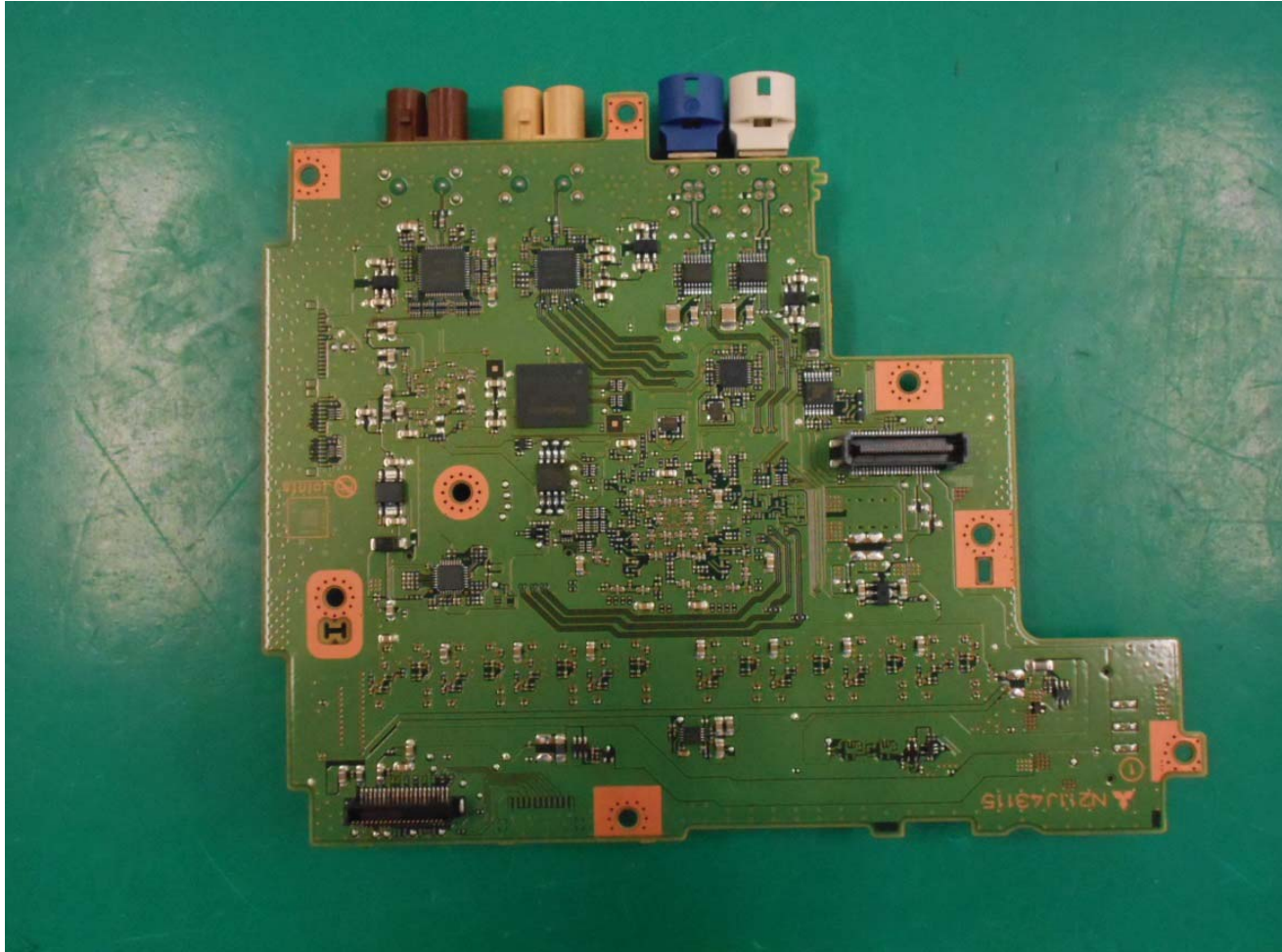
2. PCB-NAVI S-side
