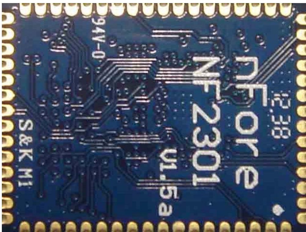
Module bottom
