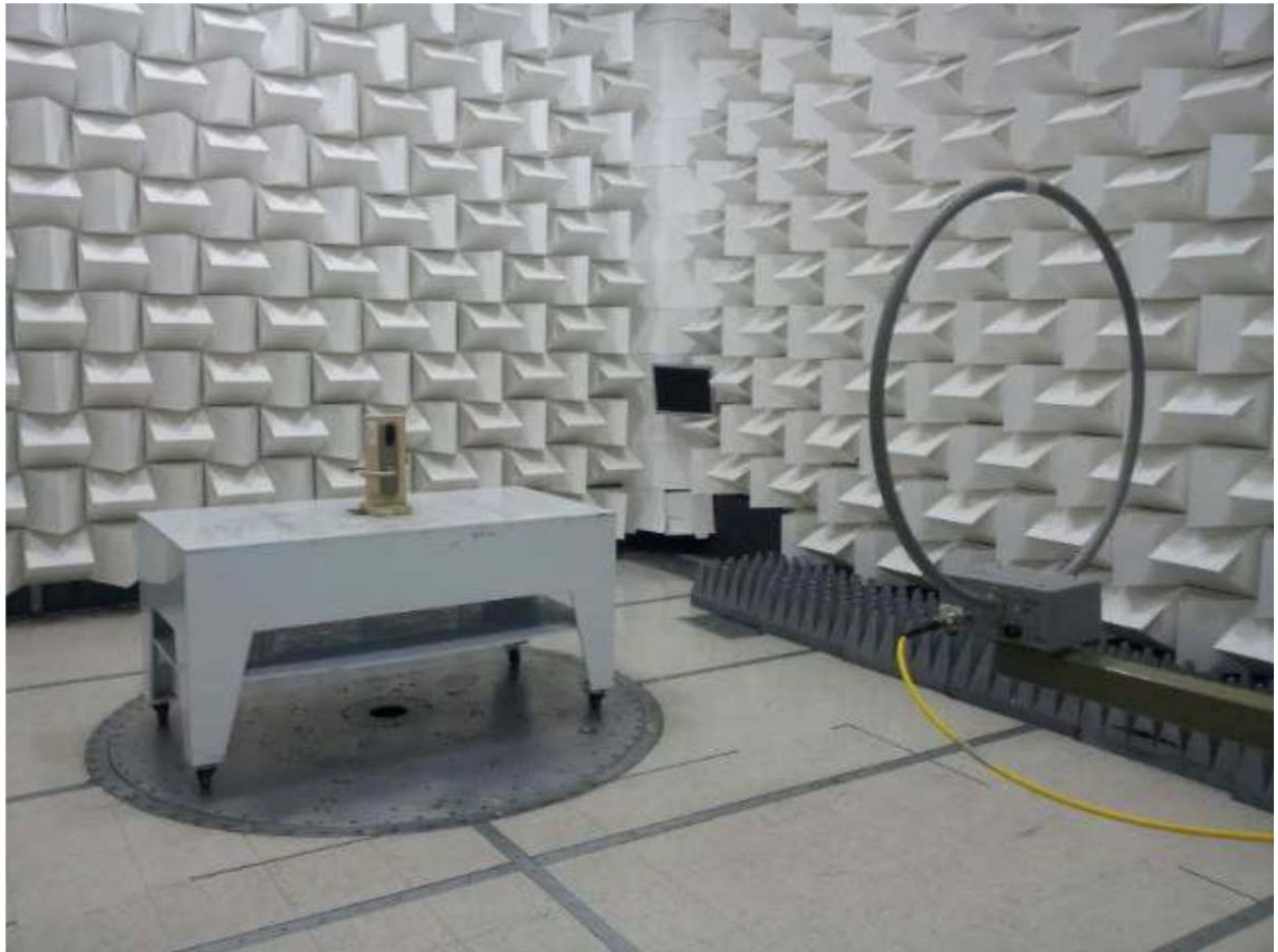
9kHz – 30MHz setup
