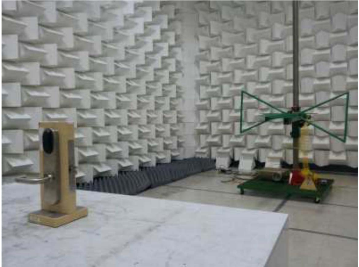
30MHz – 1000MHz setup
