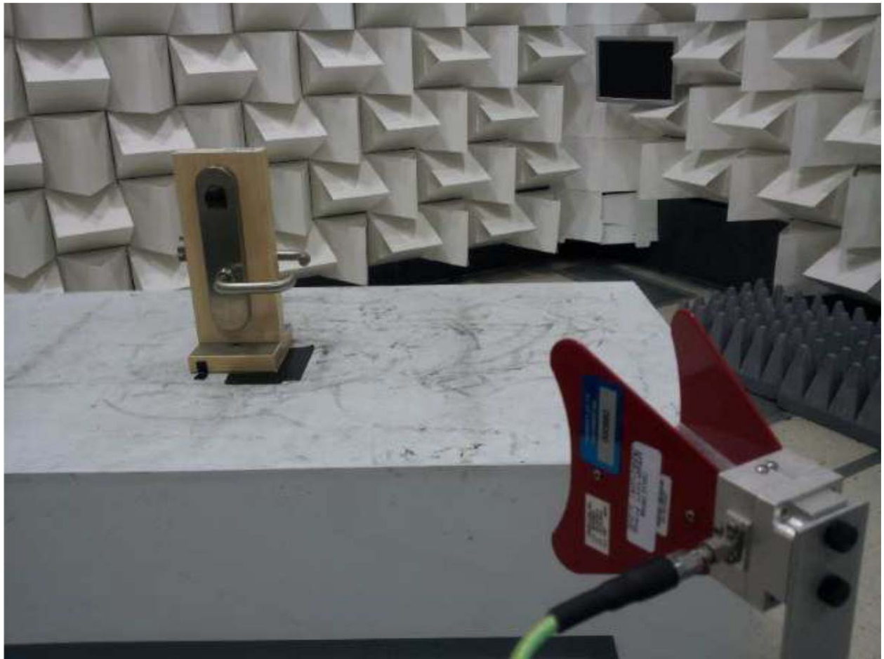
18000MHz – 26000MHz setup
