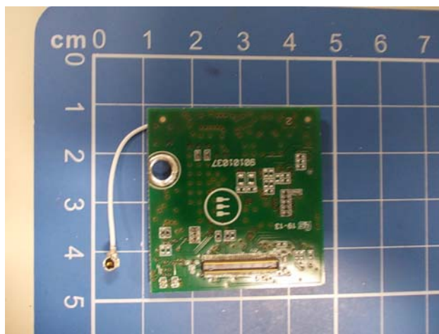
Telit GSM module bottom side
