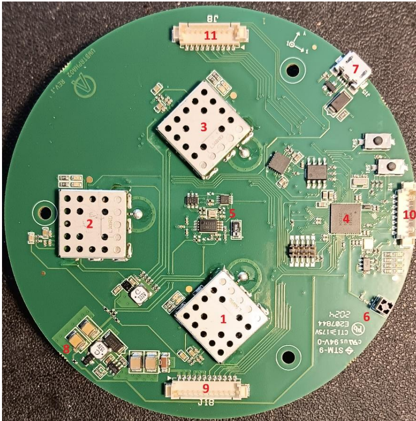
Figura 2. Bottom Side Module
