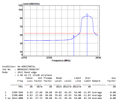
11n_HT(20M)_TX_CH_01_Horizontal-Avg
