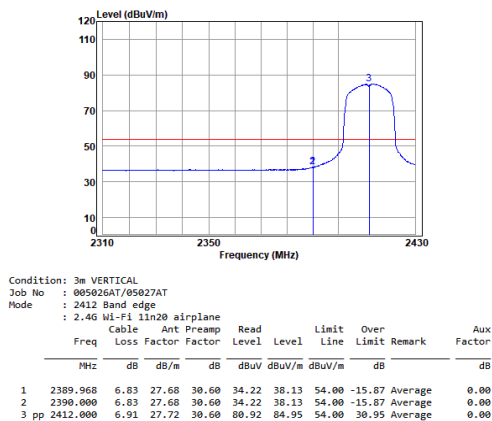
11n_HT(20M)_TX_CH_01_Vertical-Avg
