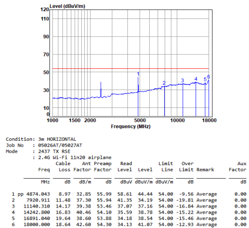
11n_20M_TX_CH_06_Horizontal-Avg
