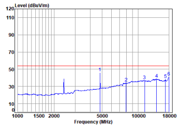
11n_20M_TX_CH_01_Horizontal-Avg
