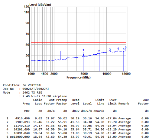
11n_20M_TX_CH_11_Vertical-Avg
