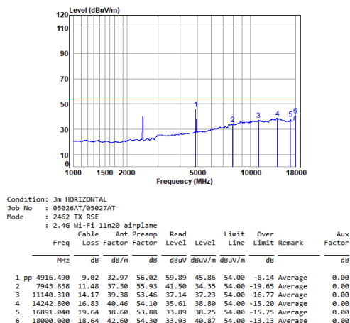
11n_20M_TX_CH_11_Horizontal-Avg
