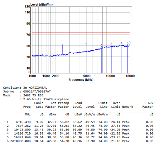
11n_20M_TX_CH_11_Horizontal-Peak
