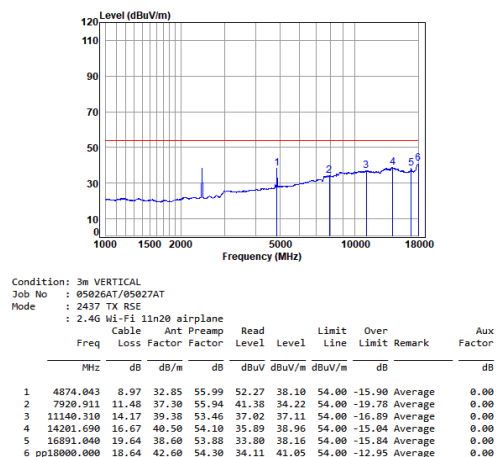
11n_20M_TX_CH_06_Vertical-Avg
