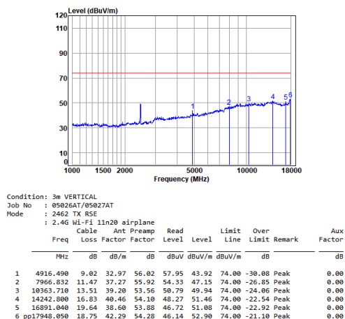
11n_20M_TX_CH_11_Vertical-Peak
