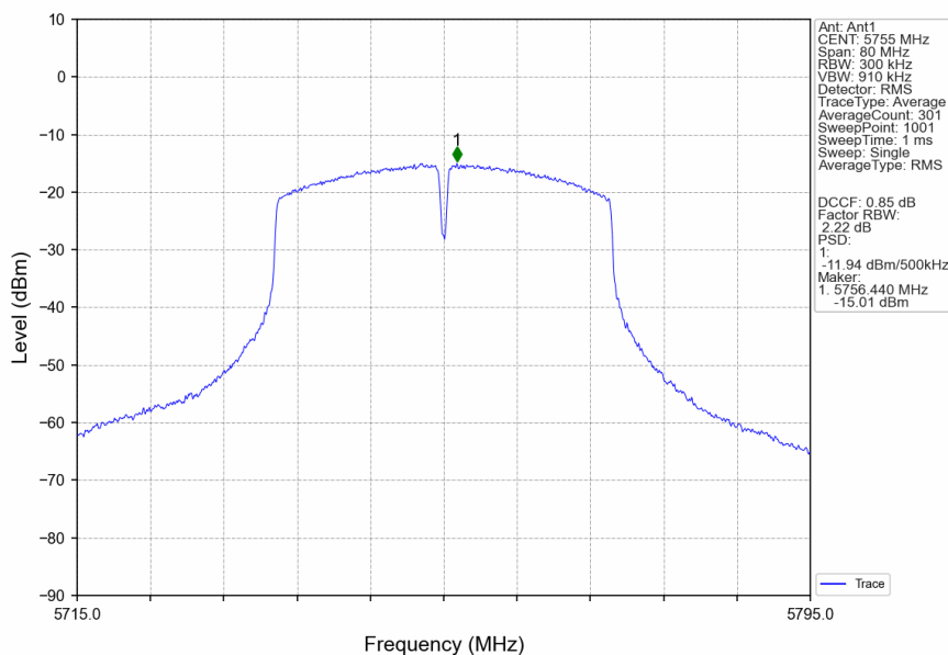
802.11n(HT40)_LCH_5755MHz_Ant1_NTNV
