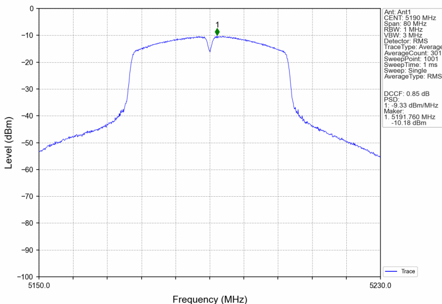
802.11n(HT40)_LCH_5190MHz_Ant1_NTNV
