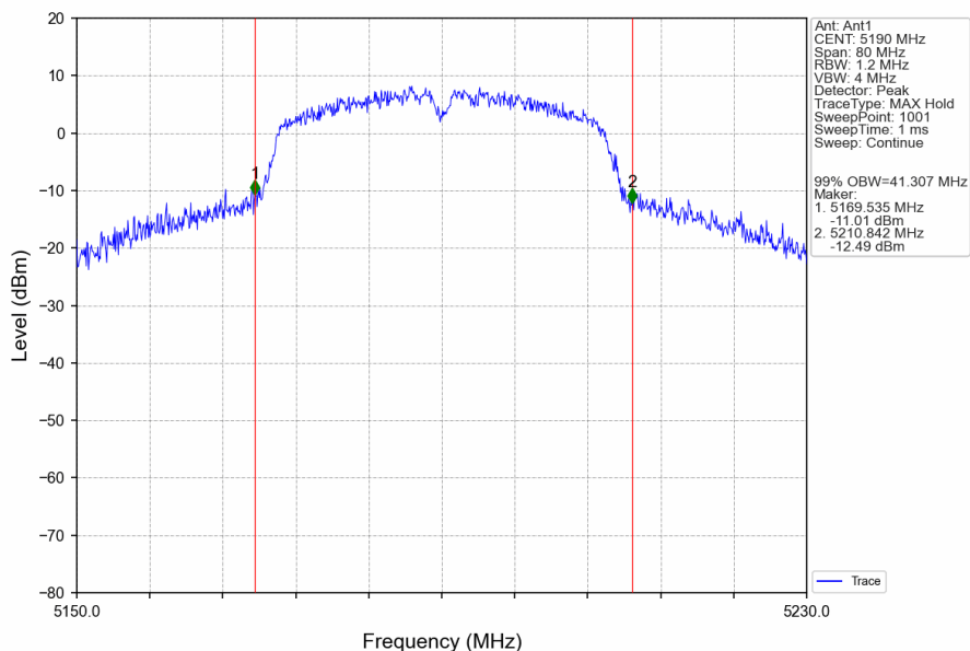
802.11n(HT40)_LCH_5190MHz_Ant1_NTNV
