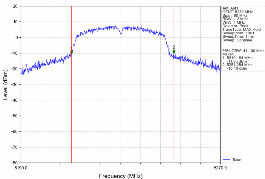
802.11n(HT40)_HCH_5230MHz_Ant1_NTNV
