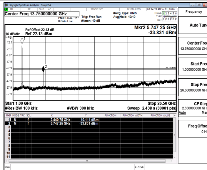
11AX40SISO_Ant2_2452_0~Reference
