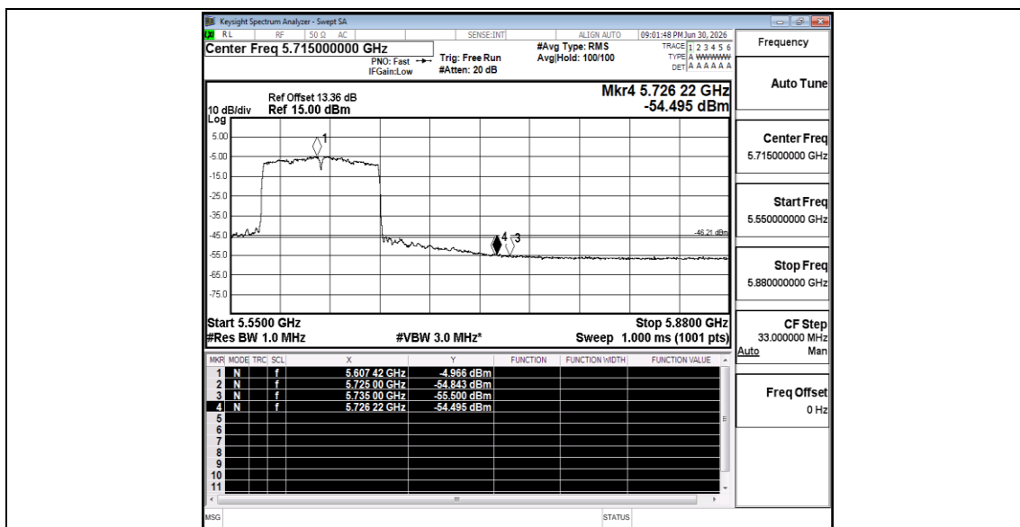
11AC80SISO Ant1 High 5610 Peak
