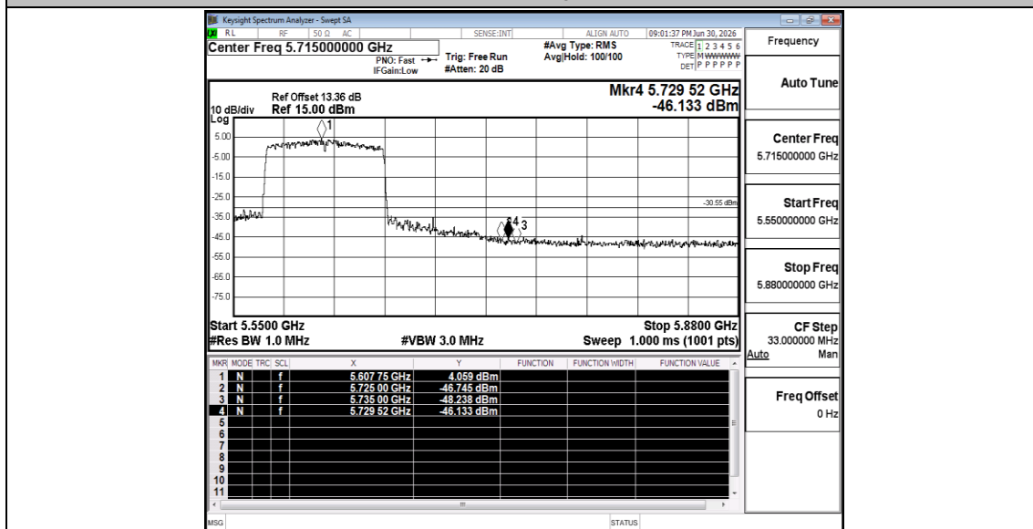
11AC160SISO Ant1 Low 5570 AV
