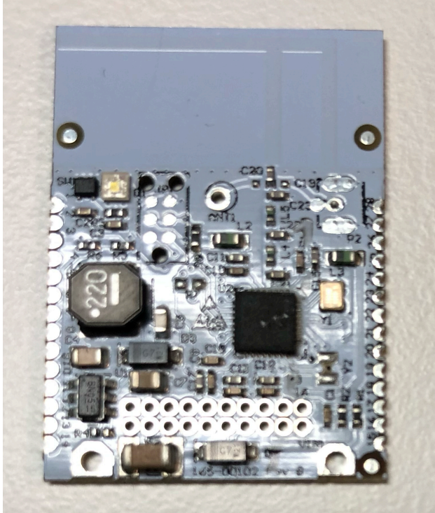
Figure 1 : EFR24CM Module
