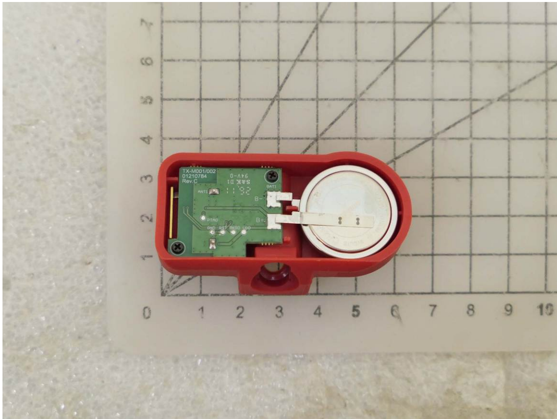
EUT-1. TX-M001
