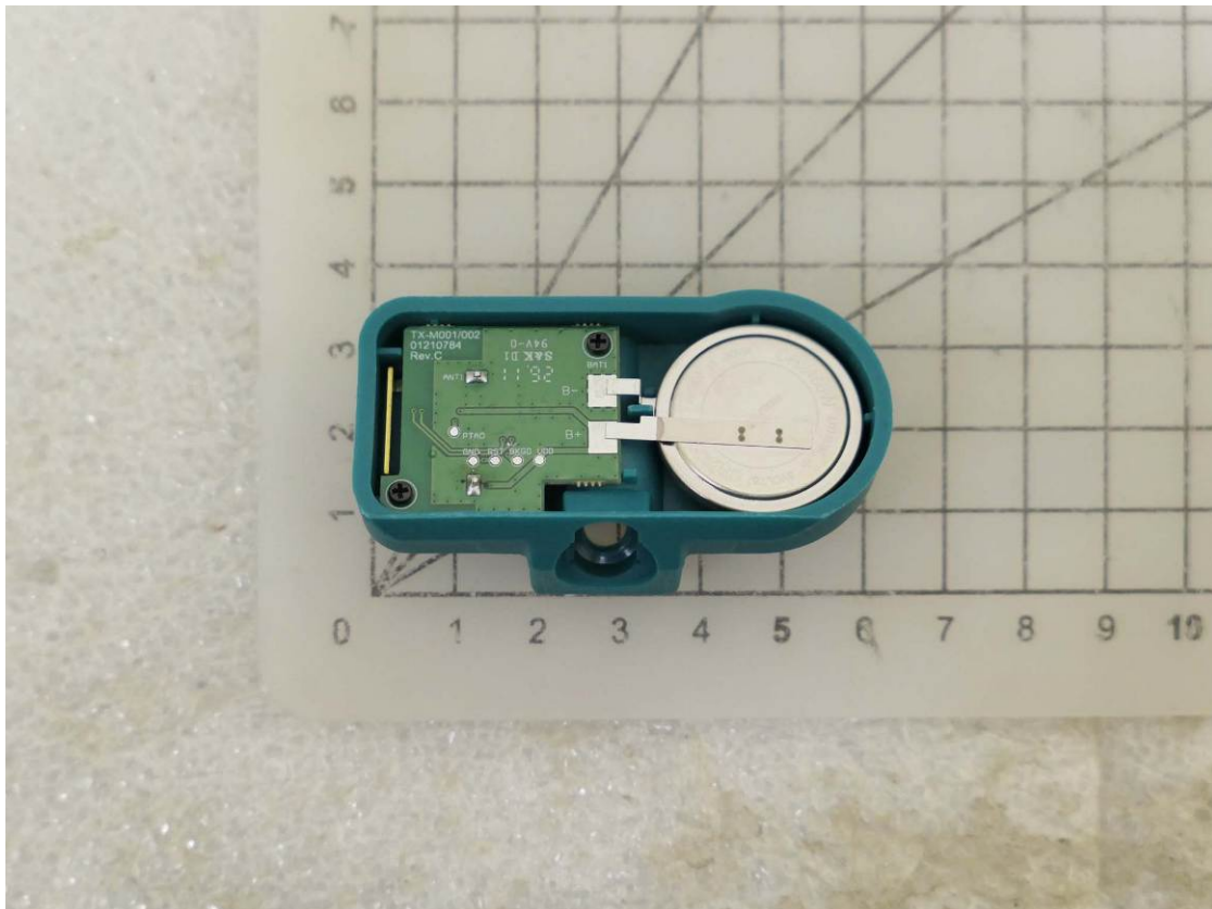
EUT-2. TX-M002
