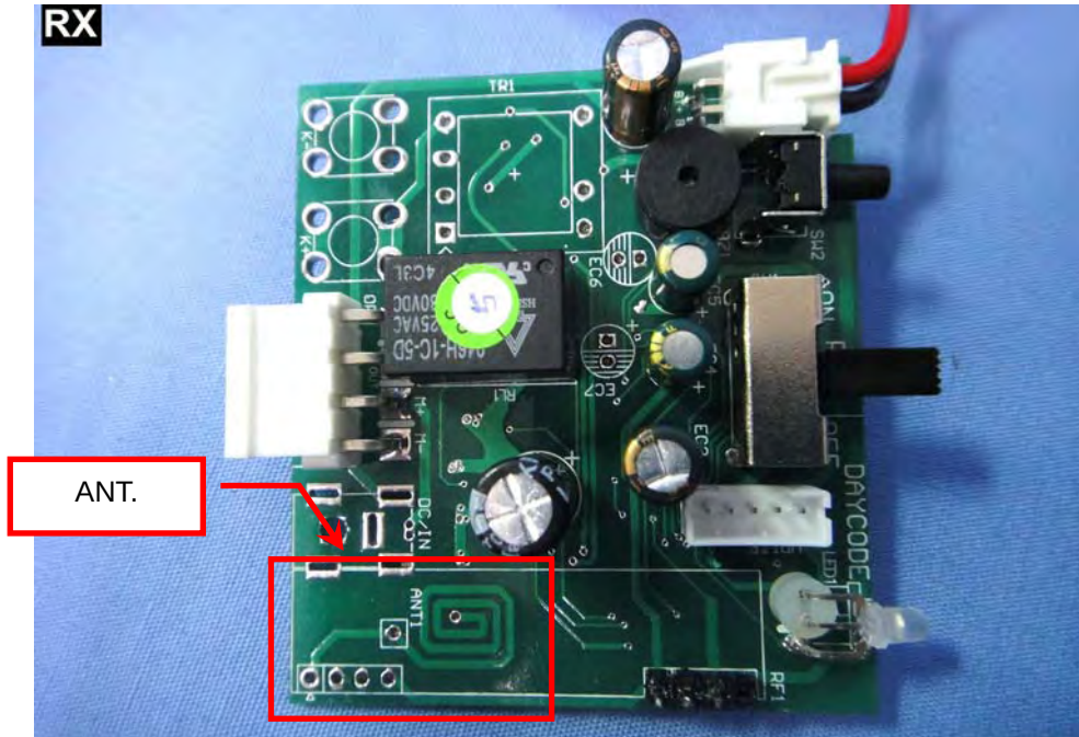
EUT Photo 7 )
