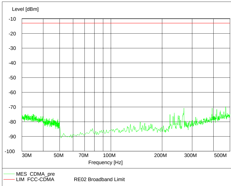
Channel 25, 30MHz~500MHz
