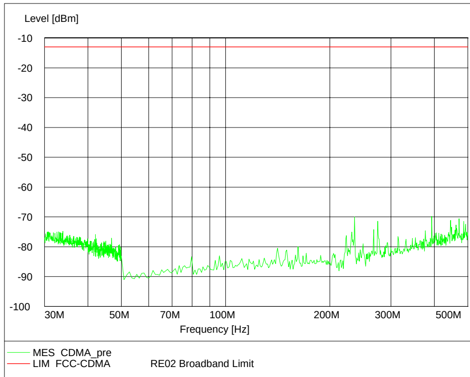
Channel 1175, 30MHz~500MHz
