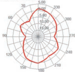
5570.000MHz E2
