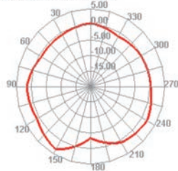
5570.000MHz E1
