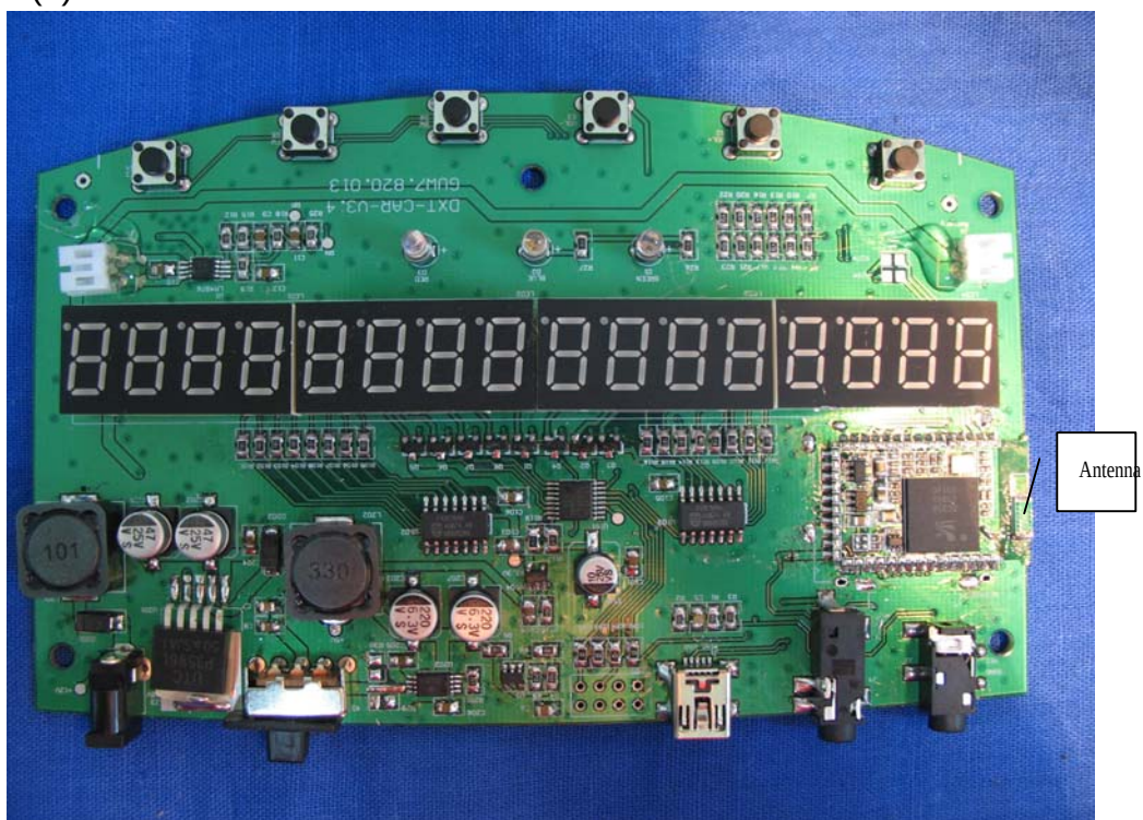
(4) EUT Photo
