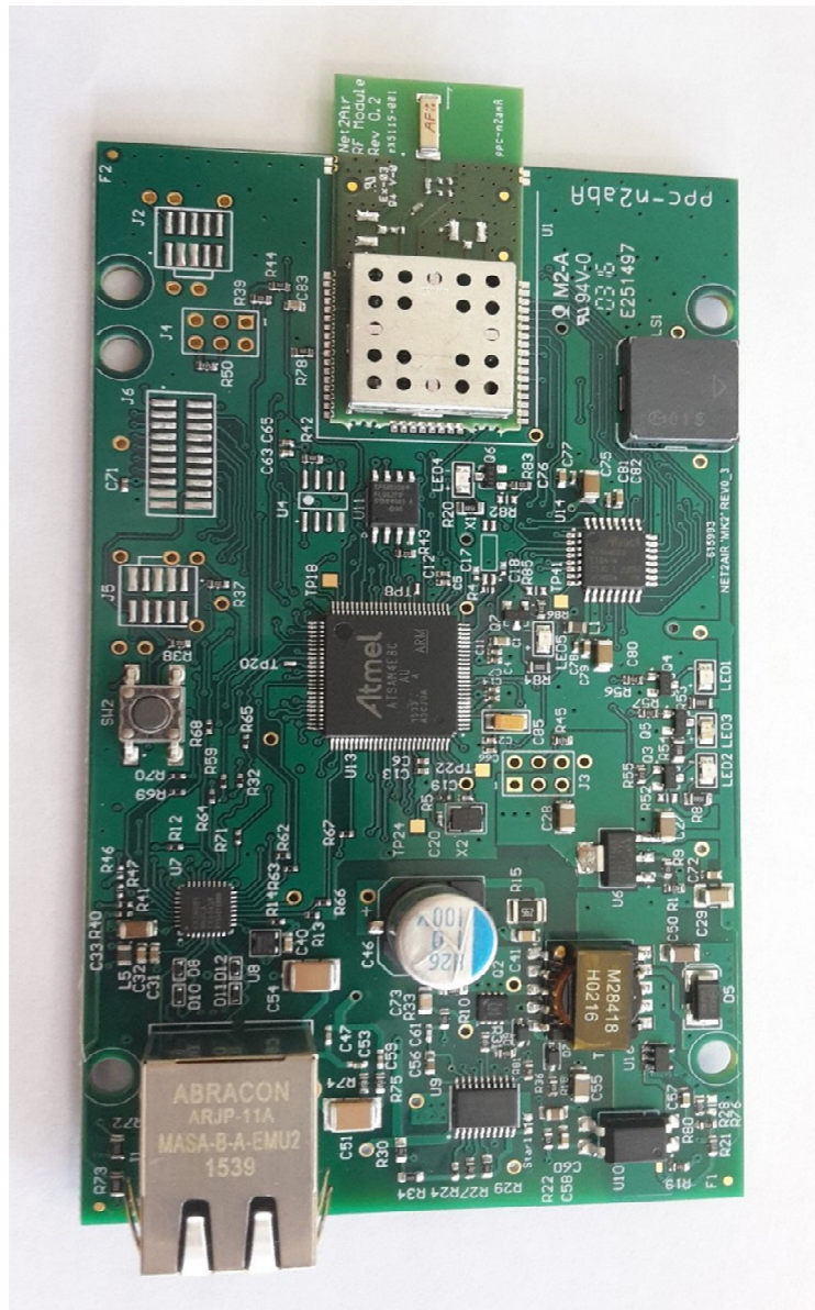
Photo 1 - Top side of PCA
