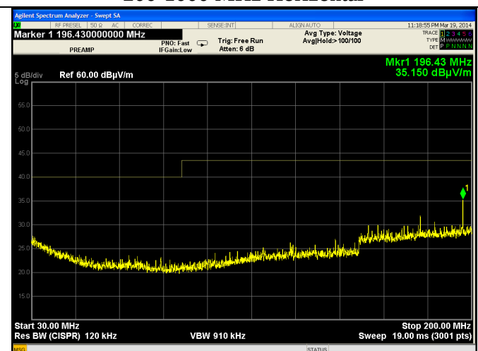
30-200 MHz Horizontal
