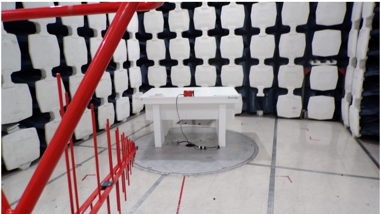
30-1000MHz
