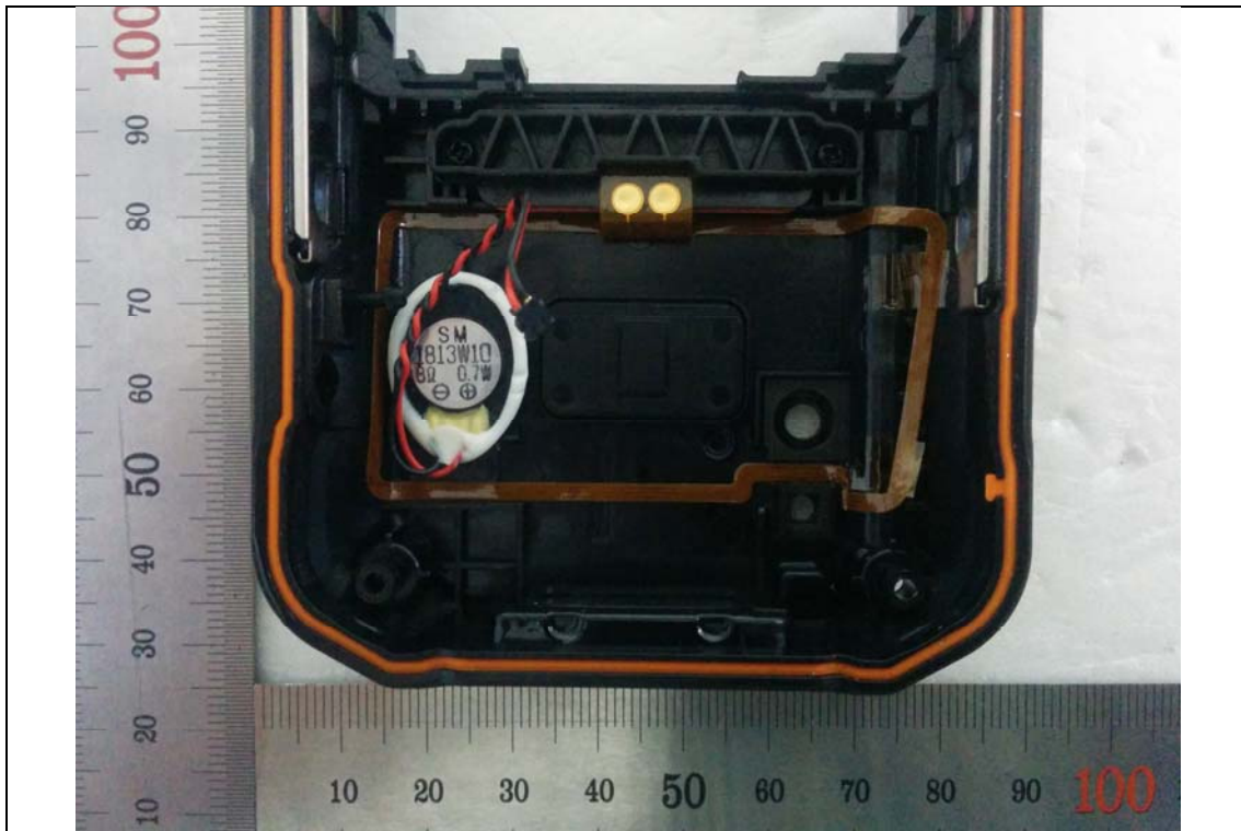
<NFC Antenna>
