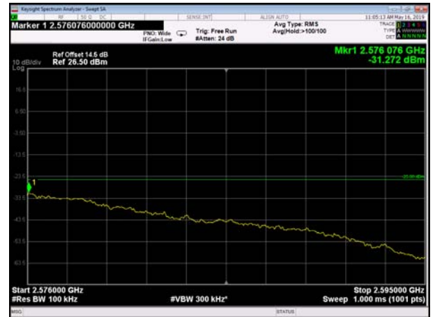
FDD07_20MHz_2560_QPSK_fullIRB_ExtraBan ds_Range_2576~2595 39
