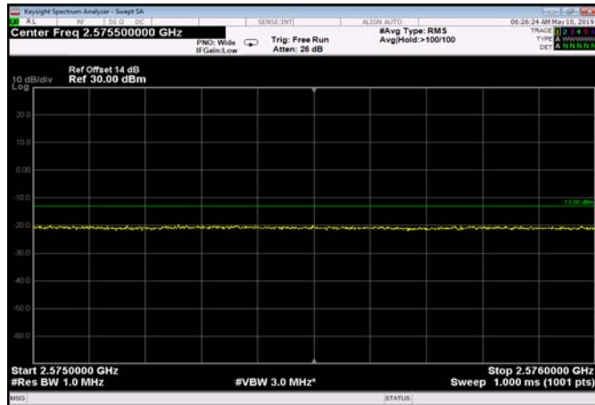
FDD07_20MHz_2560_QPSK_fullIRB_ExtraBan ds_Range_2575~2576
