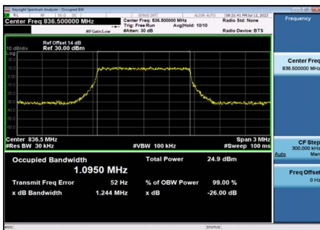
FDD26_(Part 22&RSS-132) _MidRange_3_836.5_QPSK
