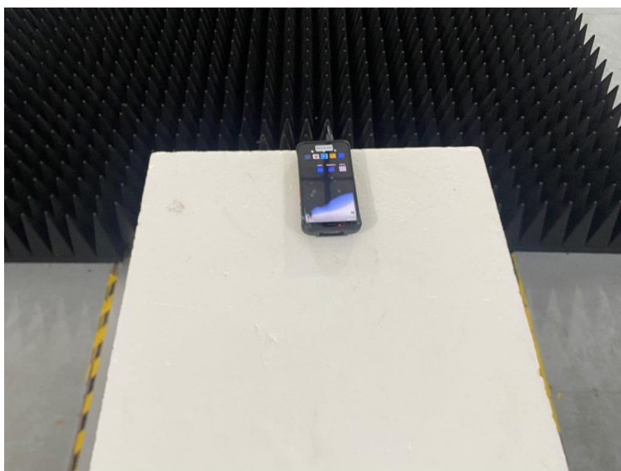
Close-up-BT/WIFI
