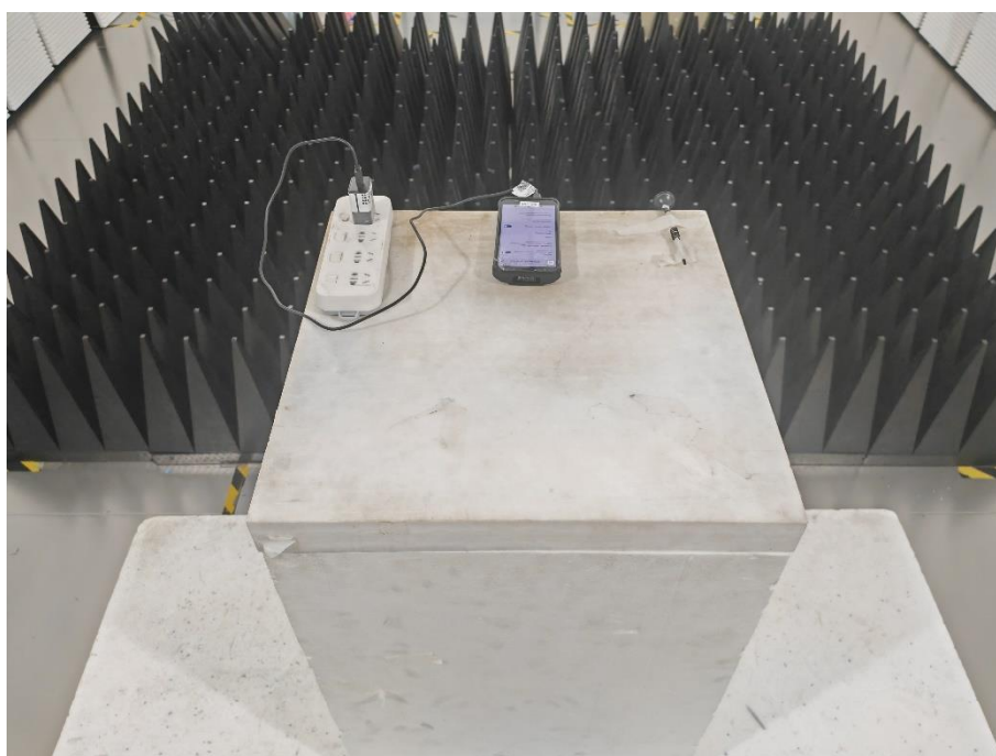
RSE-Close-up-RF
