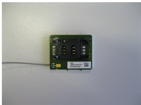
Fig. 11: Telit module - BOTTOM side
