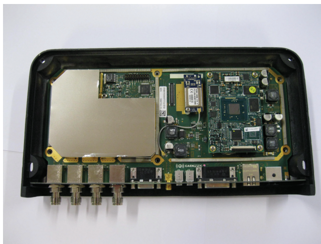
Fig. 3: R4301PXWIFI - TOP side
