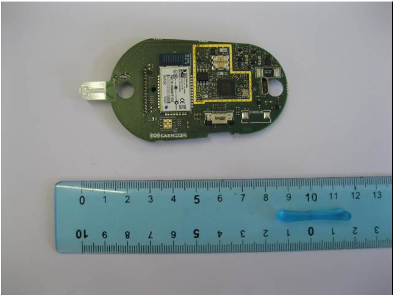
Fig. 2: PCB Bottom Side
