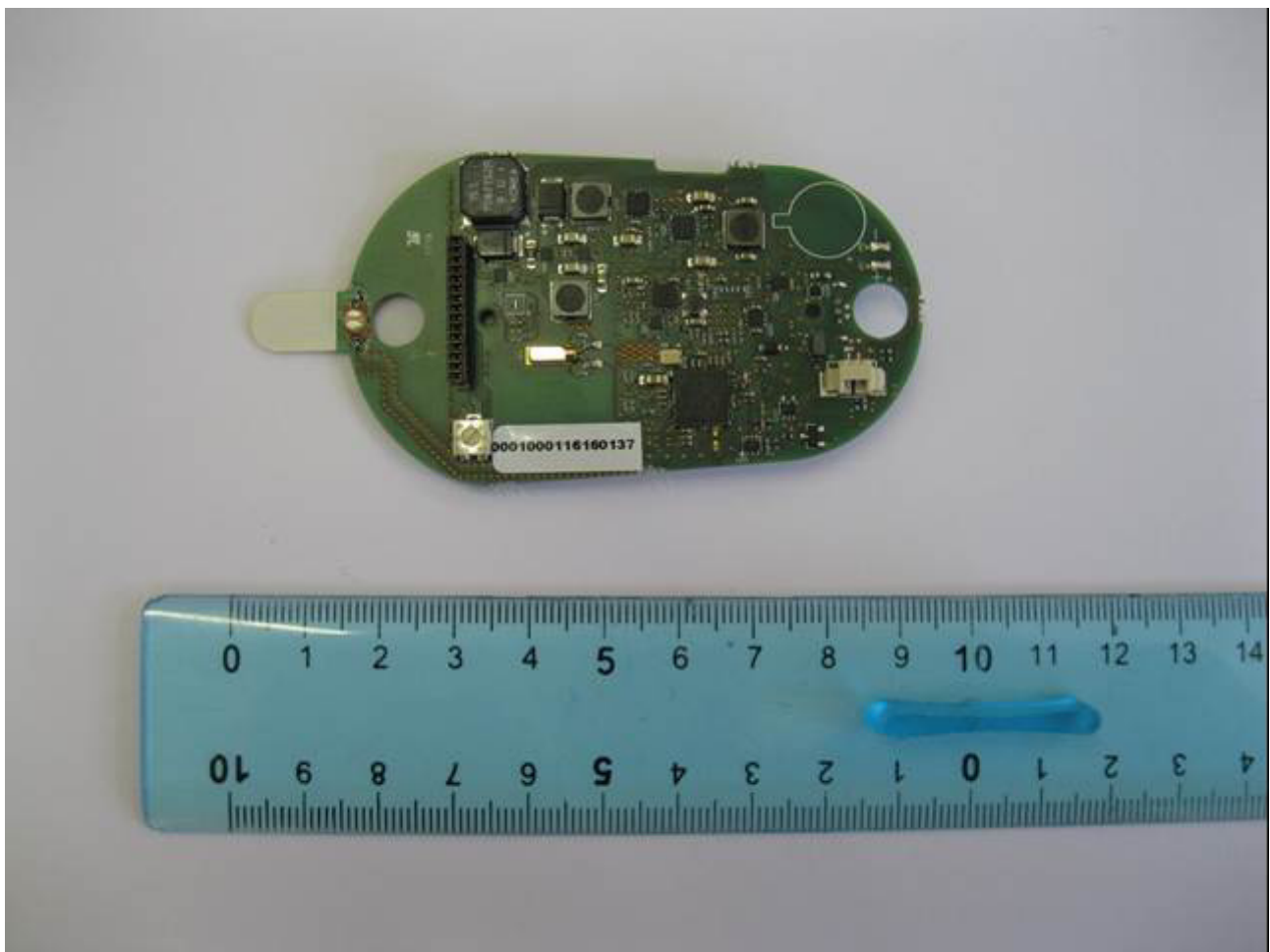
Fig. 1: PCB Top Side
