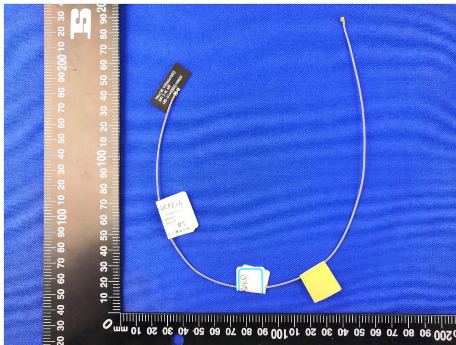
Antenna-Vista 120/Vista 120S
