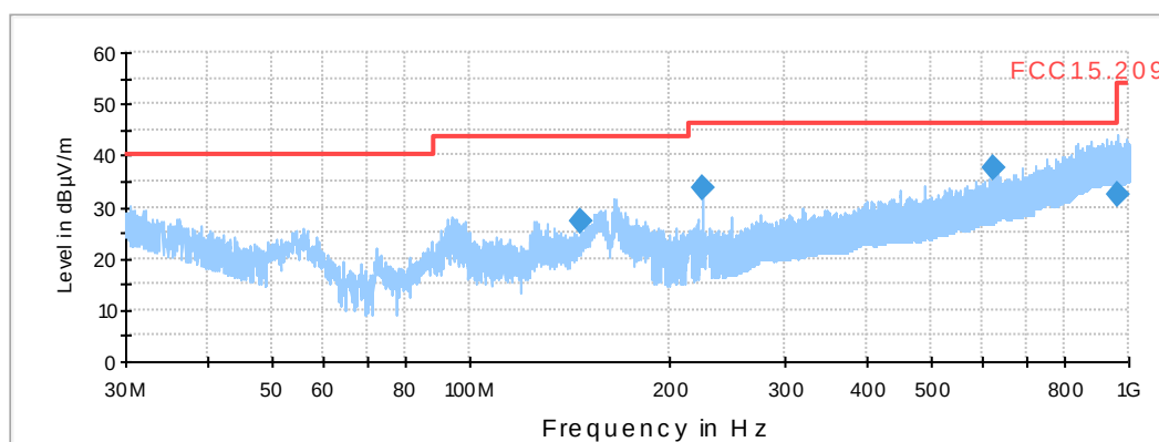
01_FCC15.209_hor+vert_KP0
