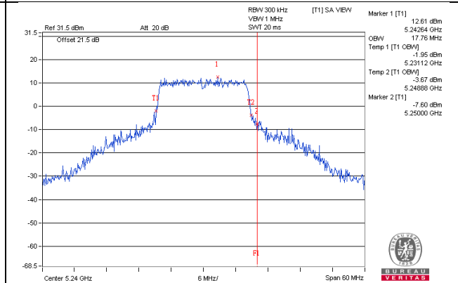
802.11ac(VHT20)_Chain1 / CH48
