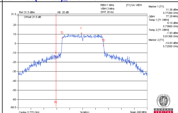
802.11ac(VHT80)_Chain1 / CH155
