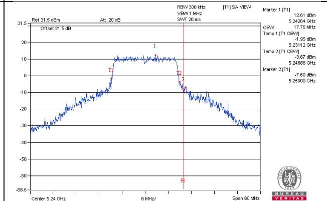
802.11ac(VHT20)_Chain1 / CH48
