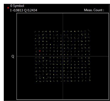
256QAM
