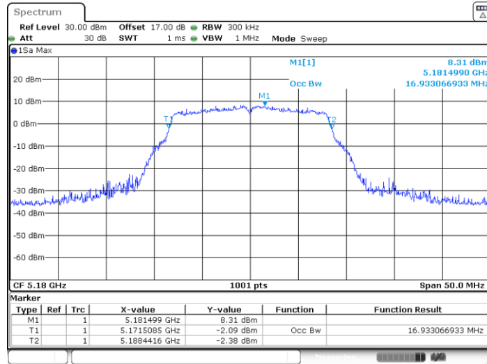
11A-CDD_Ant1_5180
