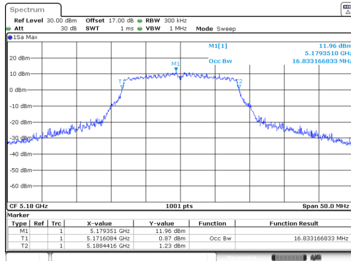
11A-CDD_Ant2_5180
