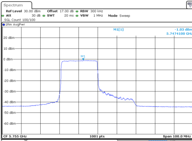
11AX40 5755MHz Partial RU242/61 MIMO Ant1
