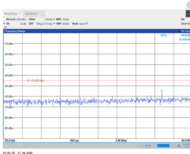
Band41-20MHz-QPSK-39750-1RB#0-Range2:0.15~30MHz
