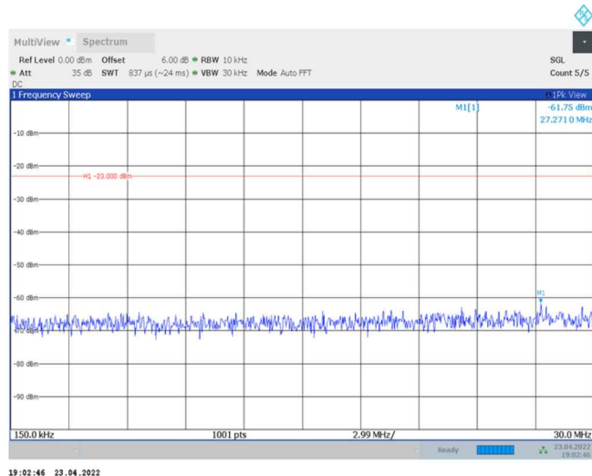
Band42-20MHz-QPSK-42190-1RB#0-Range2:0.15~30MHz
