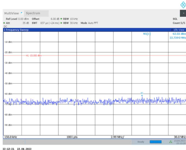
Band43-20MHz-QPSK-44690-1RB#0-Range2:0.15~30MHz
