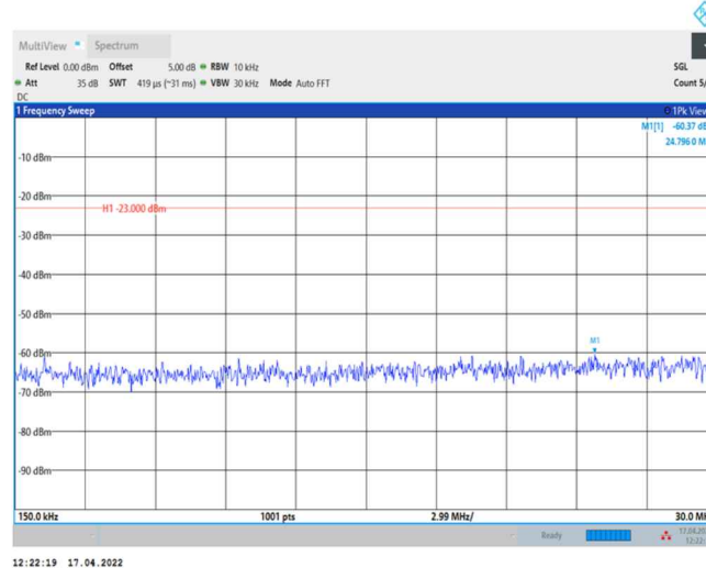
Band2-20MHz-QPSK-18700-1RB#0-Range2:0.15~30MHz
