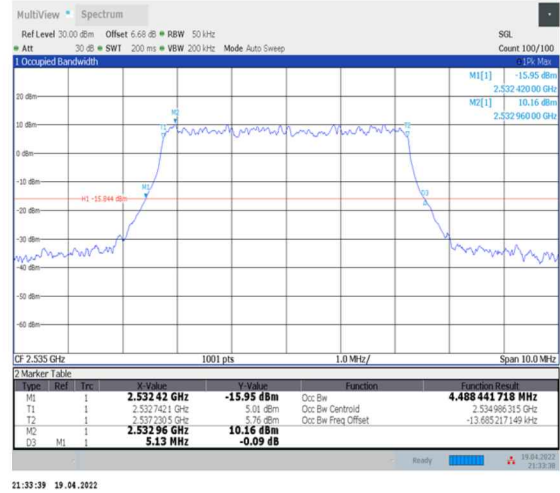
1-N7--15-5-M-5-DFT-256QAM-Outet_Full-25@0-Ant0-4.488-5.130-≤5-PASS
