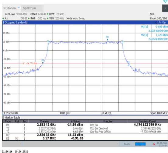
1-N7--15-5-M-6-CP-QPSK-Outet_Full-25@0-Ant0-4.474-5.170-≤5-PASS
