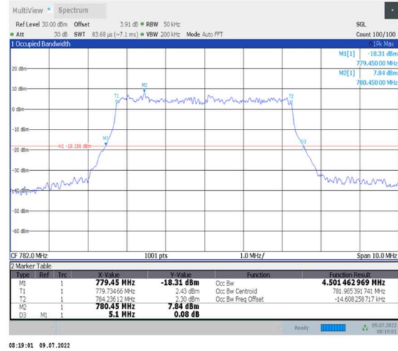
1-N13--15-5-M-9-CP-256QAM-Out Full-25@0-Ant0-4.501-5.100-≤5-PASS
