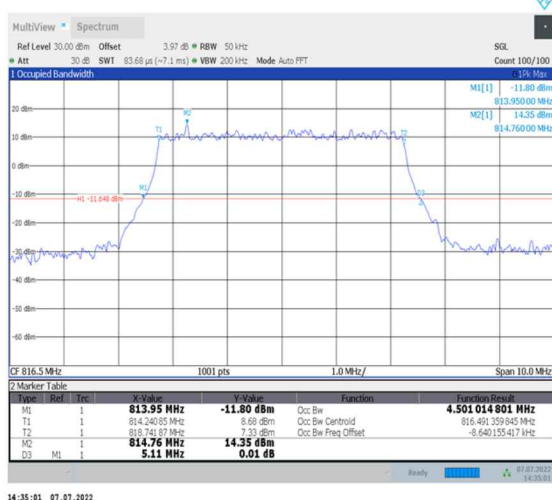
1-N26-814-824--15-5-L-1-DFT-QPSK-Outer_Full-25@0-Ant0-4.501-5.110-≤5-PASS
