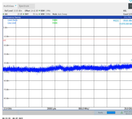
1-N26-824-849-PC3-15-20-L-1-DFT-PI2BPSK- Inner_1RB_Left-1@1-12000-20000-Ant0--39.81--13- PASS
