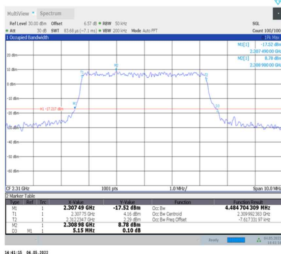
1-N30--15-5-M-7-CP-16QAM-Outer_Full-25@0- Ant0-4.485-5.150-≤5-PASS
