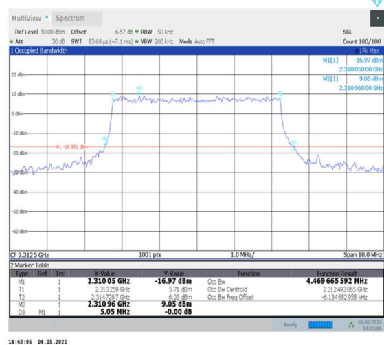
1-N30--15-5-H-6-CP-QPSK-Outer_Full-25@0-Ant0-4.47-5.050-≤5-PASS
