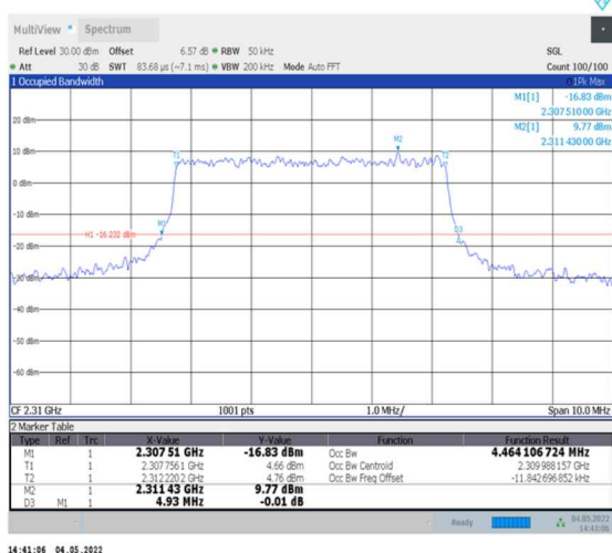
1-N30--15-5-M-6-CP-QPSK-Outer_Full-25@0-Ant0- 4.464-4.930-≤5-PASS
